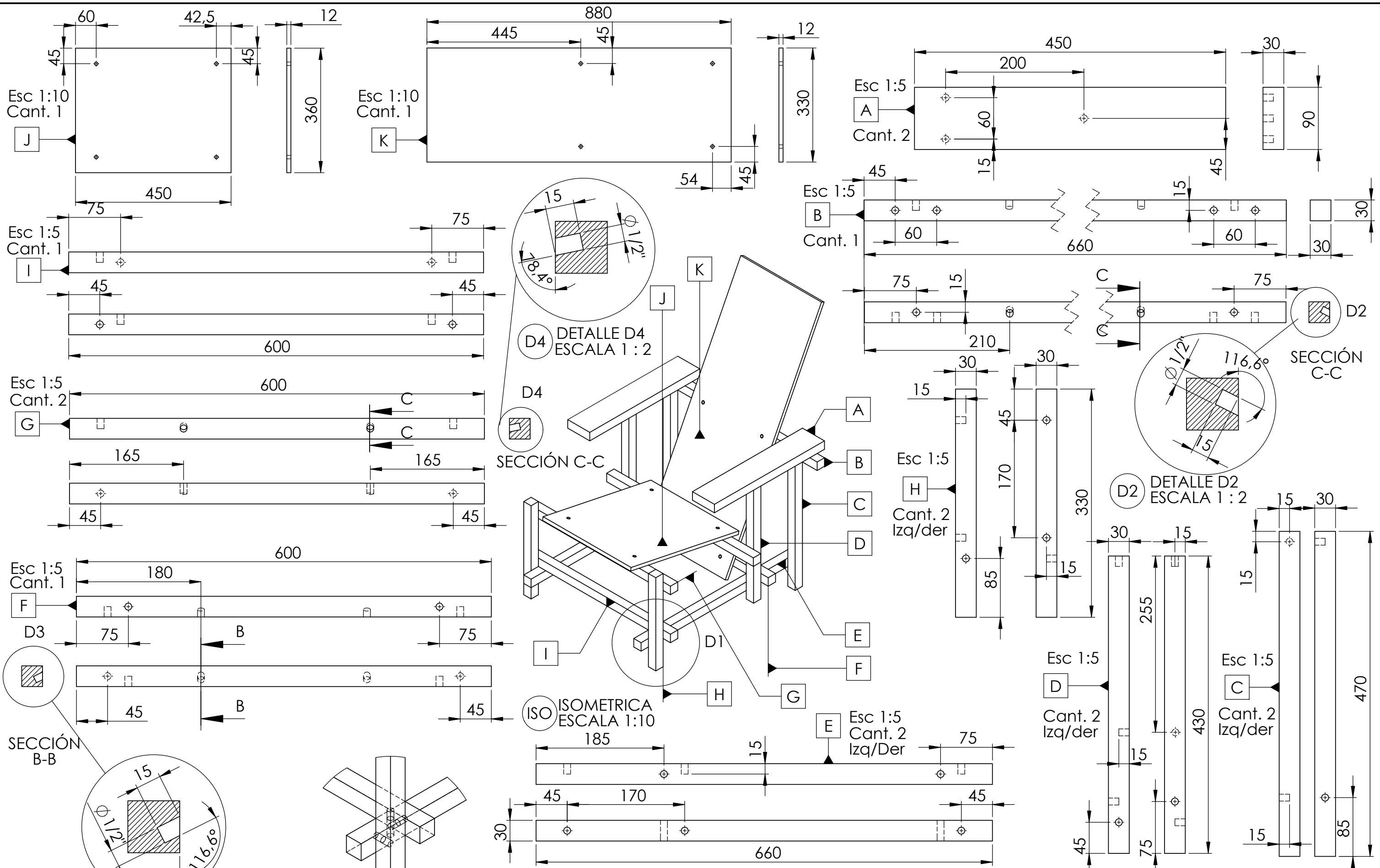
D3 DETALLE D3 ESCALA 1:2
